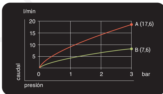
A - ROCIADOR NORMAL B - ROCIADOR AHORRADOR DUCHAFLEX
