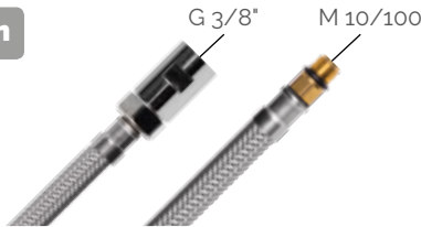
2 REF. 45941 Conexión G 3/8" de 40 cm Boquilla M 10/100 de 18 mm longitud x macho G 3/8" Hose G 3/8" 40 cm. lenght 18 mm lenght M 10/100 nozzle x G 3/8"
